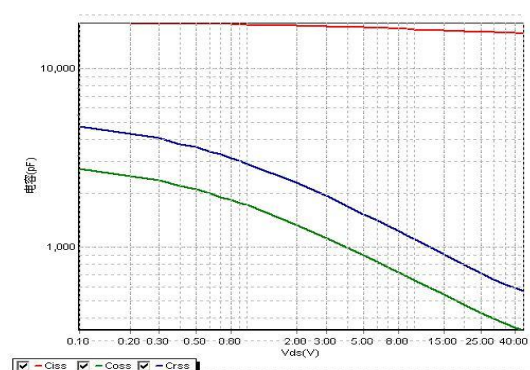
图 4 电容特性曲线
