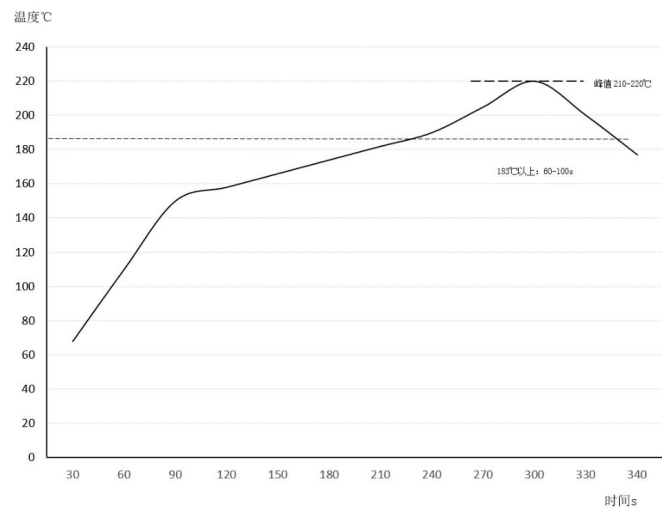
图 8 建议的回流焊曲线
