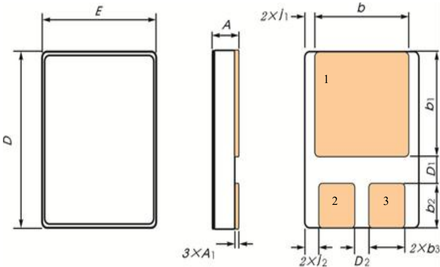
图 5 T0-257、T0-254、T0-258 外形尺寸
