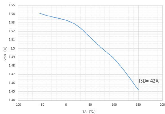
图 3 体二极管正向压降特性曲线
