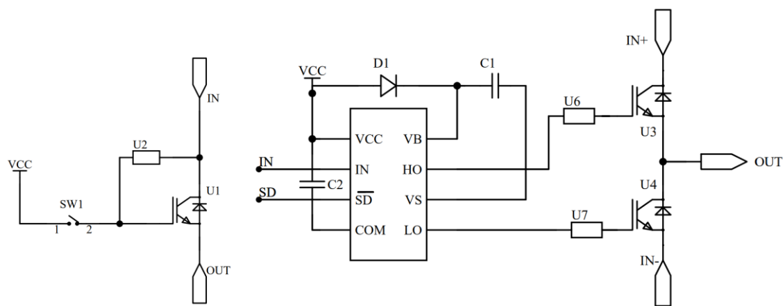
图 11 典型开关电路和驱动电路
