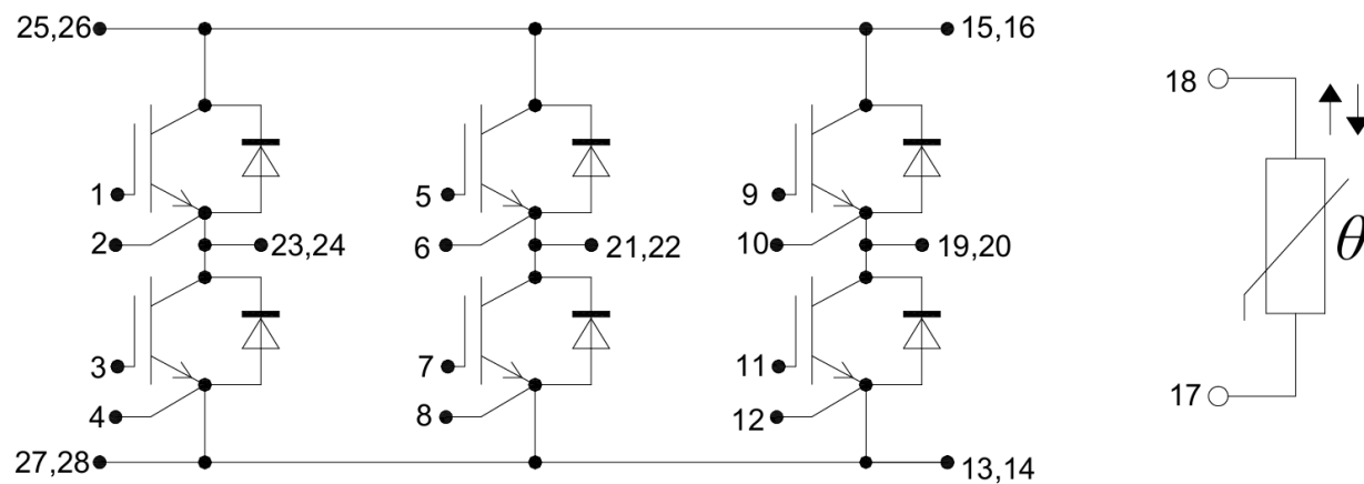
图 10 电路原理图
