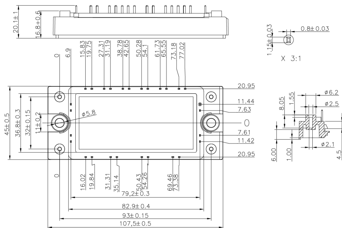
图 9 M0028A 外形尺寸图
