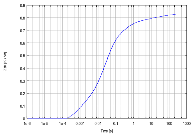
图 7 二极管瞬态热阻抗特性曲线
