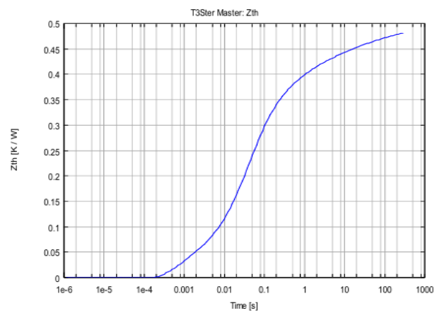
图 5 瞬态热阻抗变化曲线
