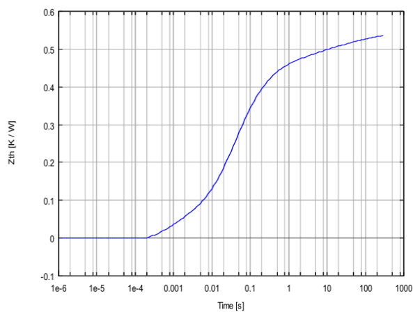
图 5 瞬态热阻抗变化曲线
