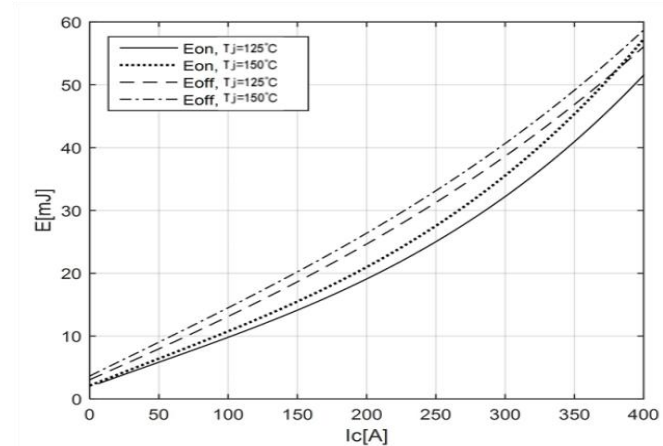
图 4 开关损耗曲线
