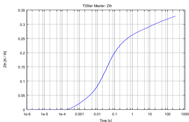
图 7 二极管瞬态热阻抗特性曲线
