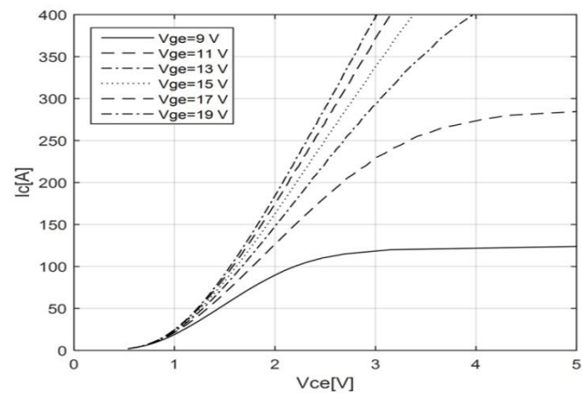
图 2 输出特性曲线
