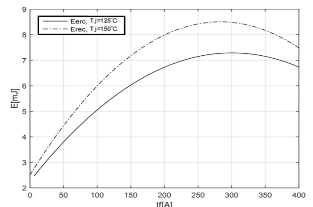
图 8 二极管开关损耗曲线
