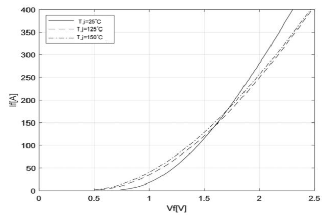
图 6 二极管正向偏压特性曲线
