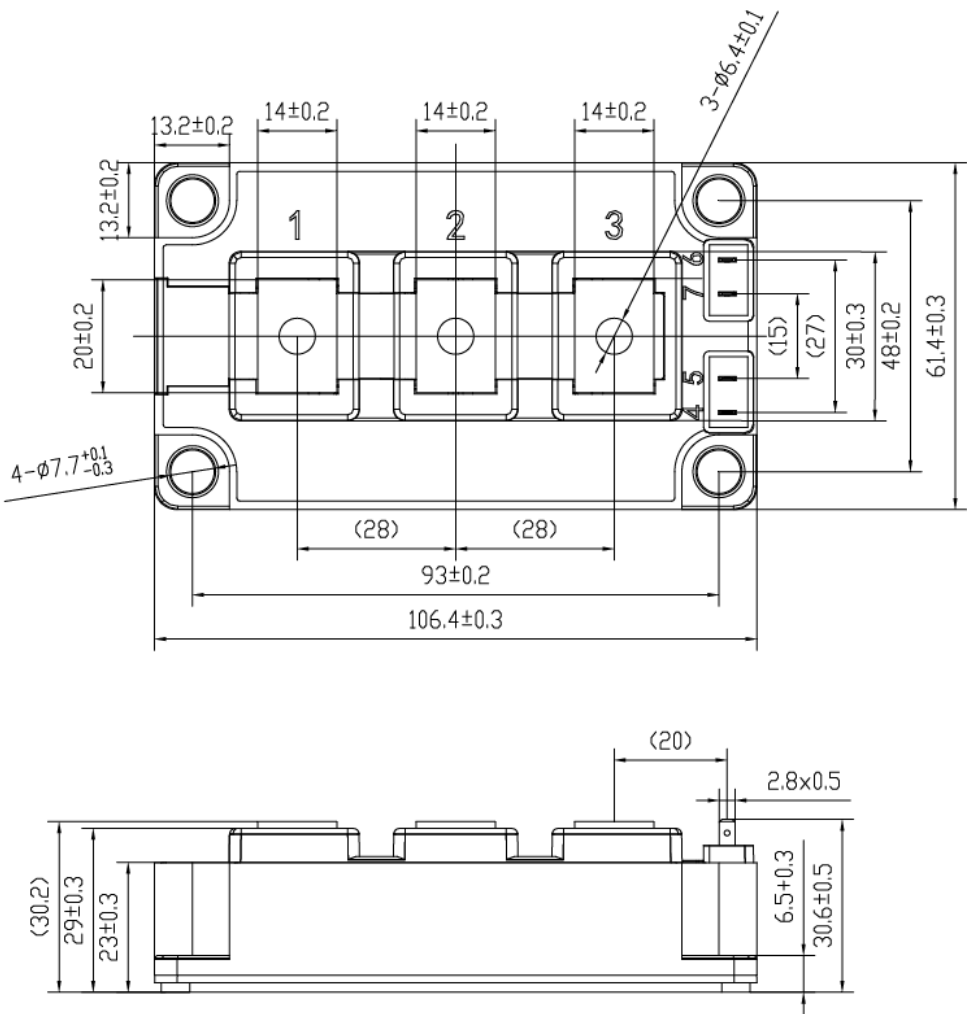
图 9 D008A 外形尺寸图
