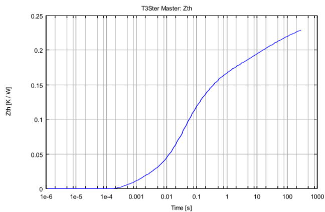
图 5 瞬态热阻抗变化曲线
