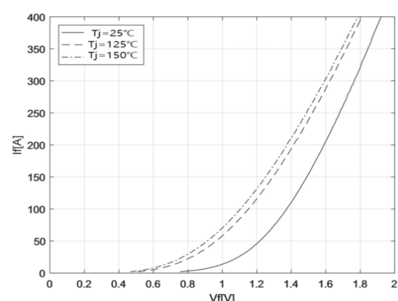
图 6 二极管正向偏压特性曲线
