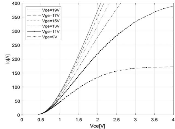
图 2 输出特性曲线
