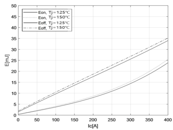
图 4 开关损耗曲线
