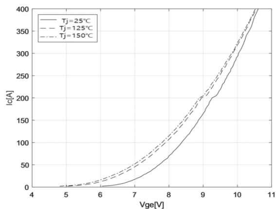
图 3 传输特性曲线
