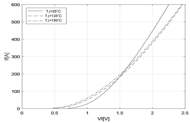
图 6 二极管正向偏压特性曲线
