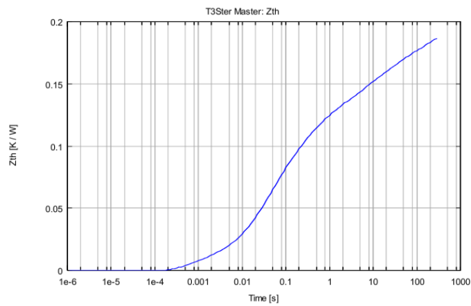
图 5 瞬态热阻抗变化曲线
