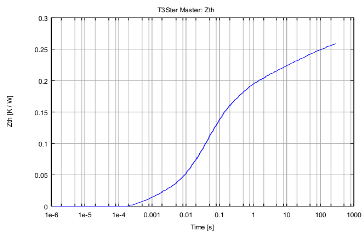
图 7 二极管瞬态热阻抗特性曲线
