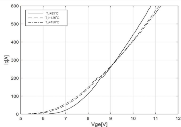
图 3 传输特性曲线
