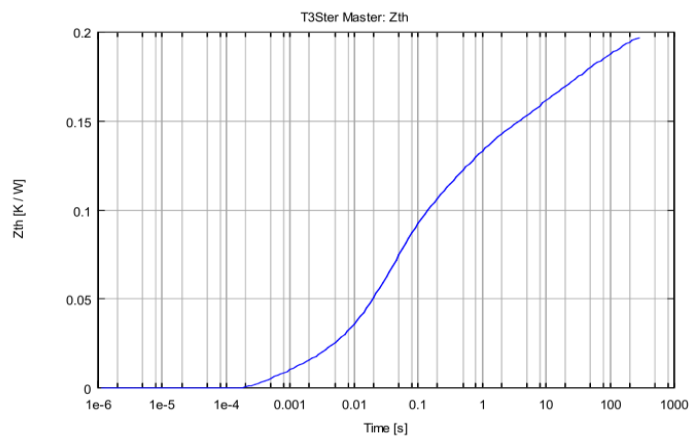
图 7 二极管瞬态热阻抗特性曲线
