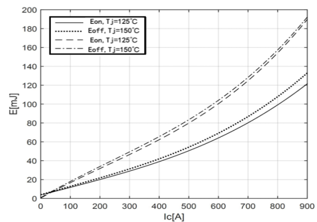
图 4 IGBT 开关损耗曲线
