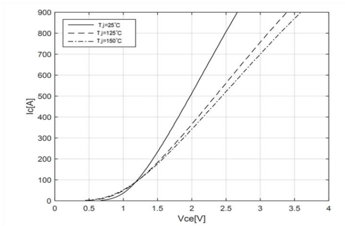
图 1 输出特性曲线
