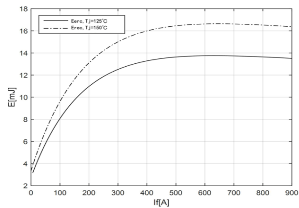
图 8 二极管开关损耗曲线
