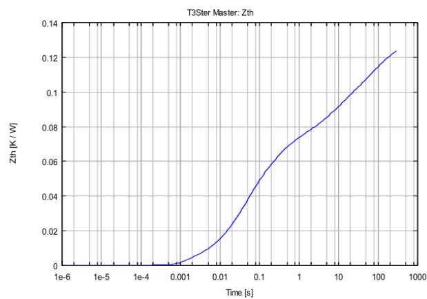
图 5 瞬态热阻抗变化曲线
