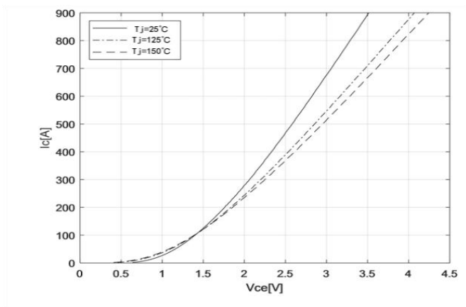
图 1 输出特性曲线
