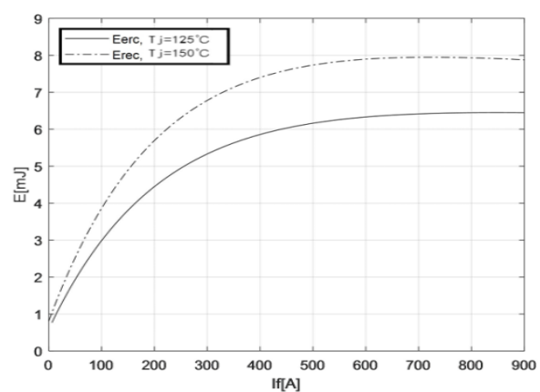
图 8 二极管开关损耗曲线
