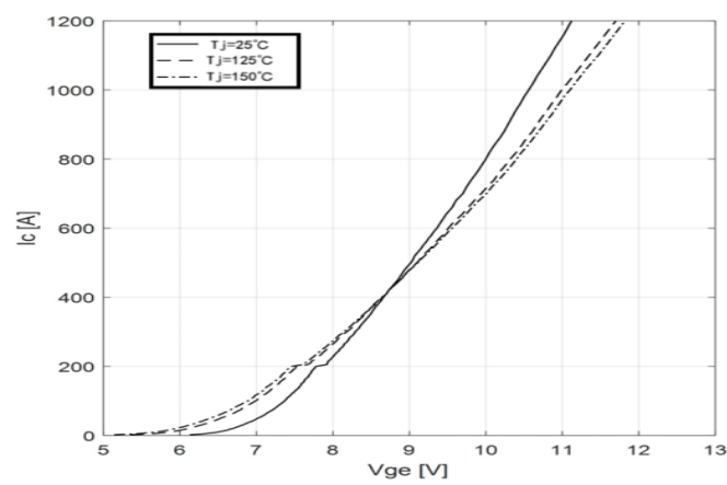
图 3 传输特性曲线
