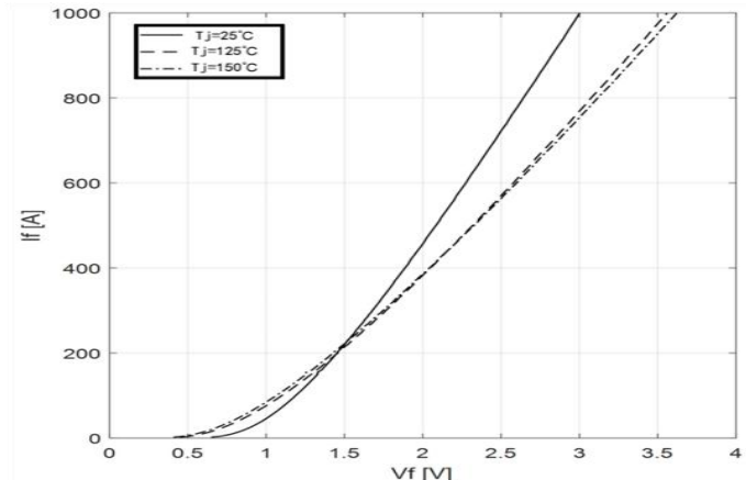
图 6 二极管正向偏压特性曲线
