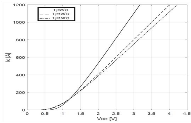
图 1 输出特性曲线
