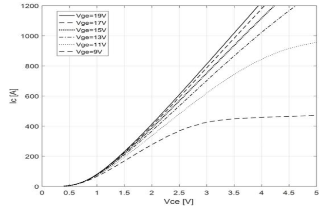
图 2 输出特性曲线
