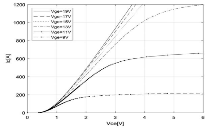
图 2 输出特性曲线
