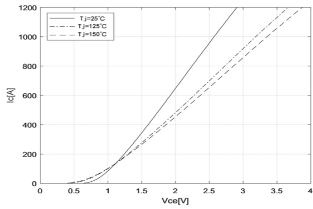
图 1 输出特性曲线
