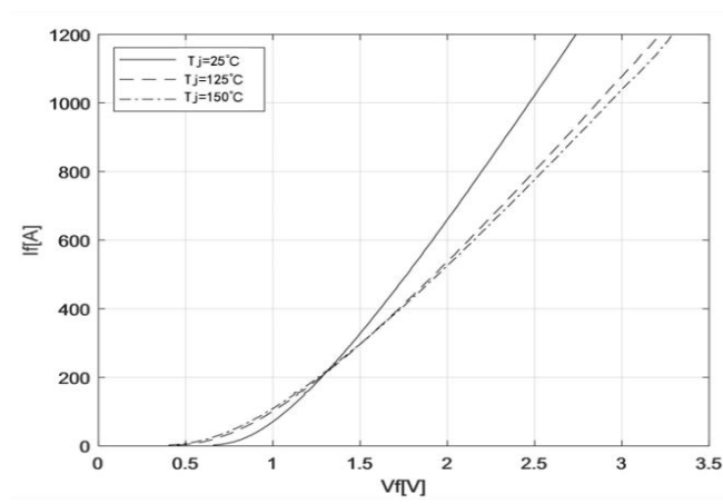
图 6 二极管正向偏压特性曲线
