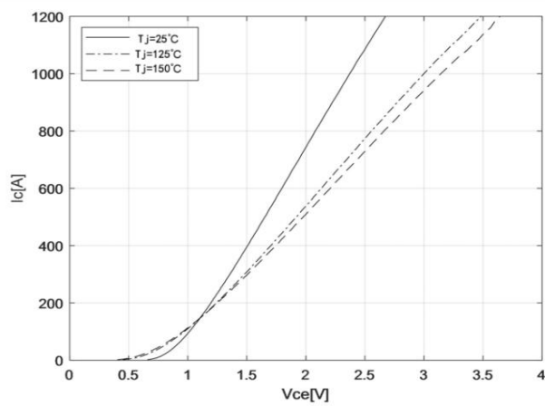
图 1 输出特性曲线
