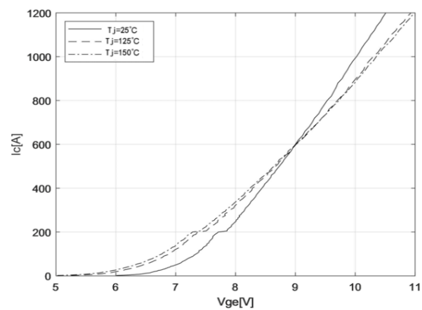
图 3 传输特性曲线
