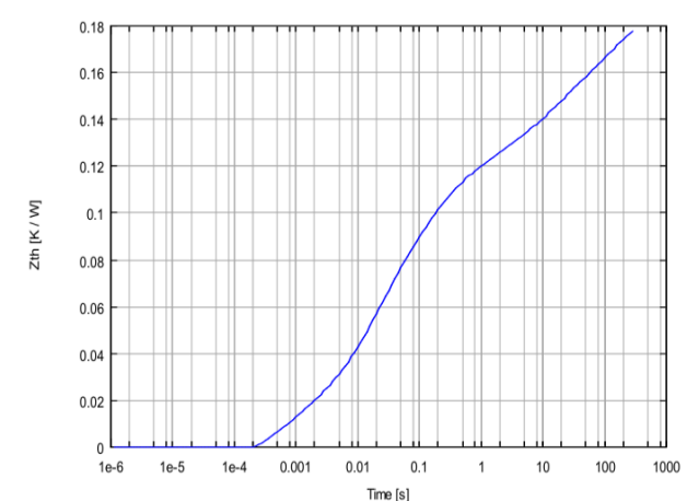
图 7 二极管瞬态热阻抗特性曲线
