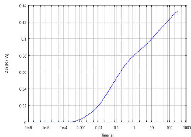
图 5 瞬态热阻抗变化曲线
