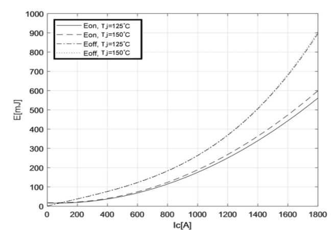
图 4 开关损耗曲线
