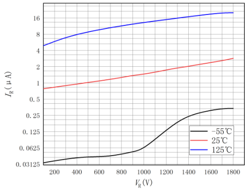
图 2 反向特性曲线
