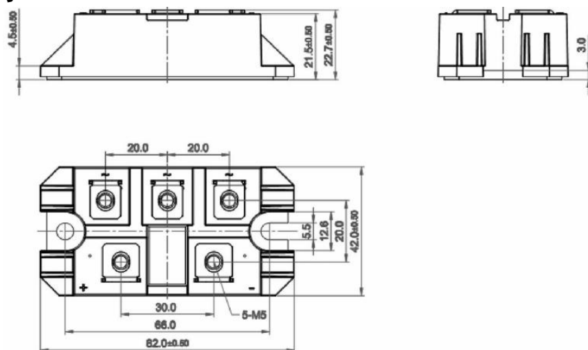
图 4 M0025A 外形尺寸
