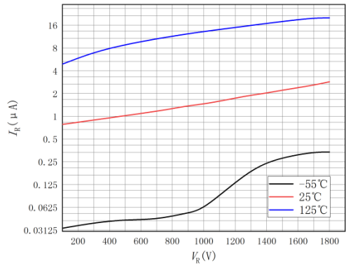
图 2 反向特性曲线
