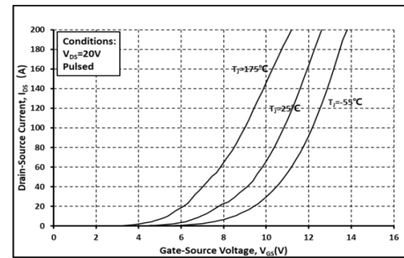
图 2 转移特性曲线
