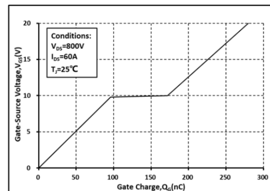
图 4 栅电荷特性曲线
