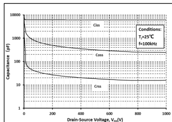
图 5 C - V_{DS} 特性曲线
