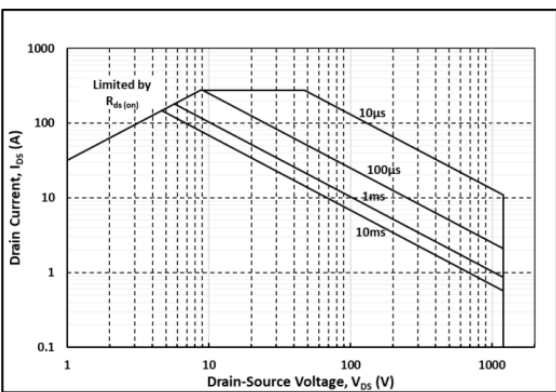
图 6 安全工作区曲线
