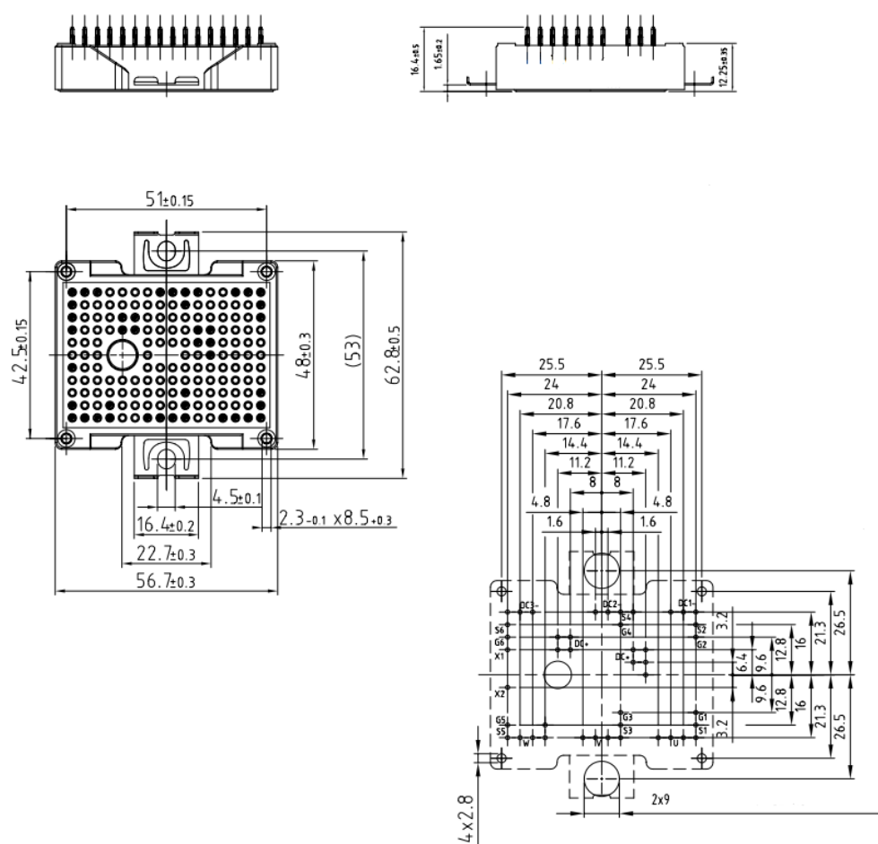
图 12 M0019A 外形尺寸图
