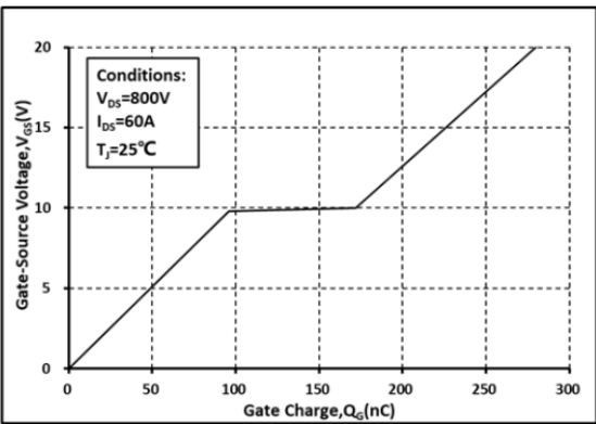
图 4 栅电荷特性曲线
