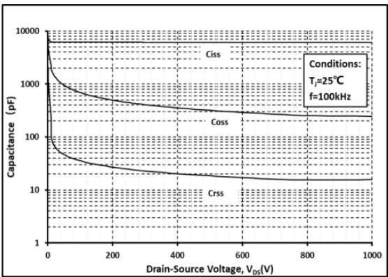
图 5 C- V_{DS} 特性曲线
