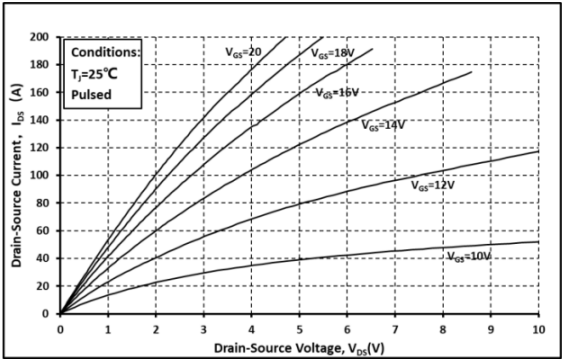
图 1 输出特性曲线
