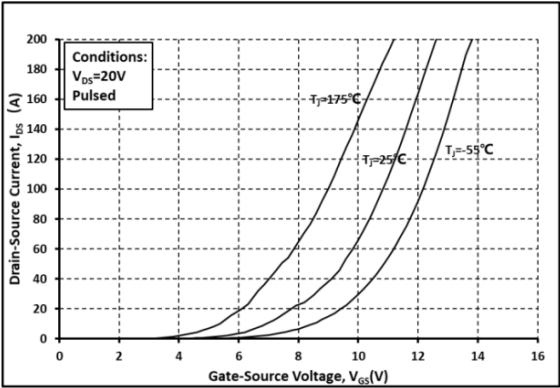
图 2 转移特性曲线
