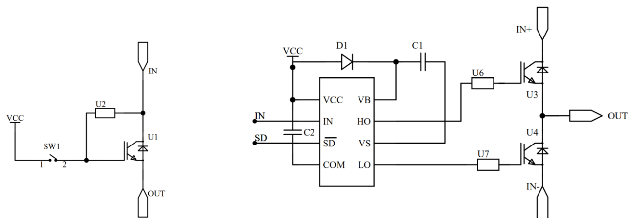
图 13 典型开关电路和驱动电路
