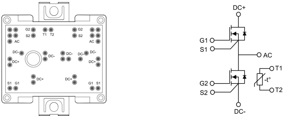
图 13 引线端子连接图
