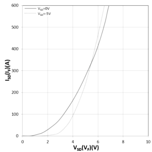
图 4 T_J=175^{\circ}C , 体二极管特性曲线
