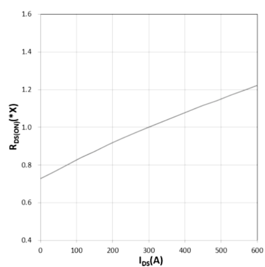
图 6 R_{DS(on)} 随 I_D 的变化曲线
