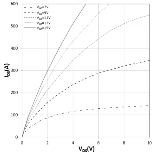
图 1 输出特性曲线
