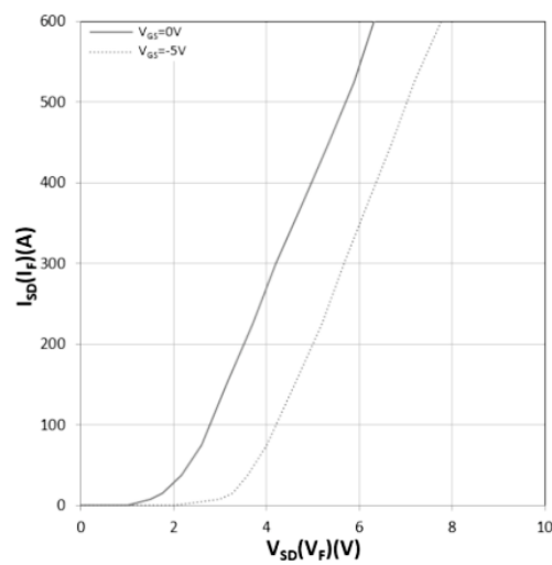
图 3 体二极管特性曲线
