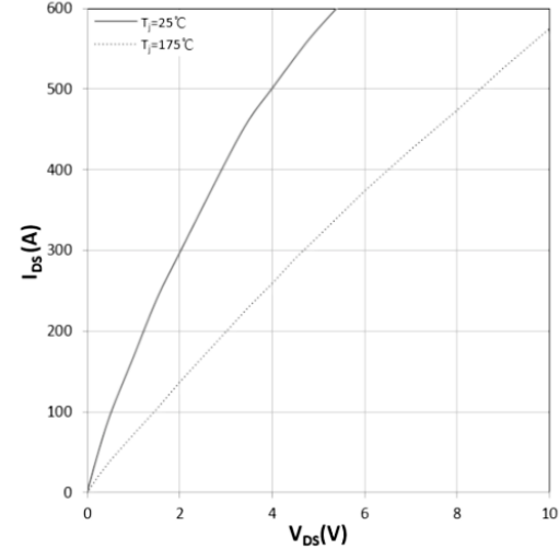
图 2 不同温度输出特性曲线
