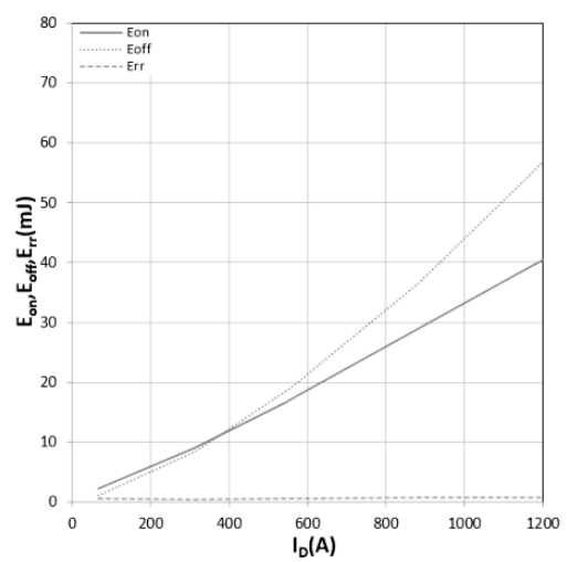
图 11 E_{on} , E_{off} , E_{rr} 随 I_{DS} 的变化曲线
