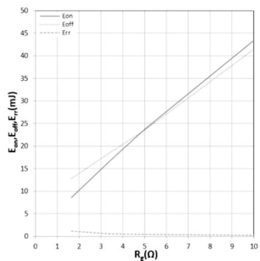
图 9 E_{on} , E_{off} , E_{rr} 随 R_g 的变化曲线
