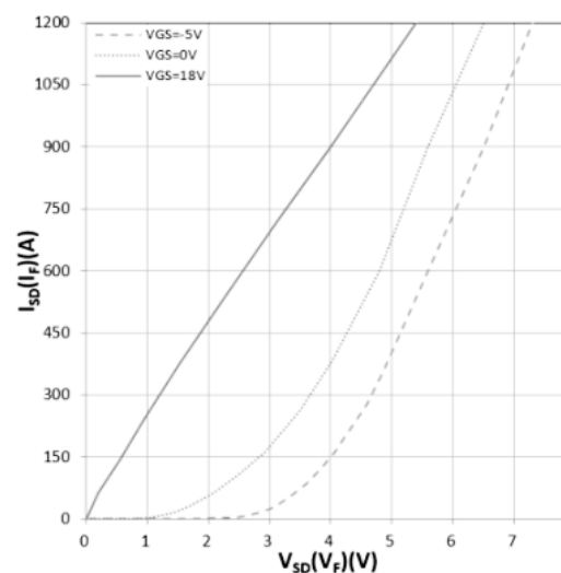
图 4 I_F 随 V_F 的变化曲线
