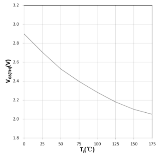
图 8 V_{GS(th)} 随 T_j 的变化曲线
