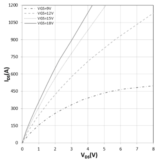
图 1 I_D 随 V_{DS} 的变化曲线
