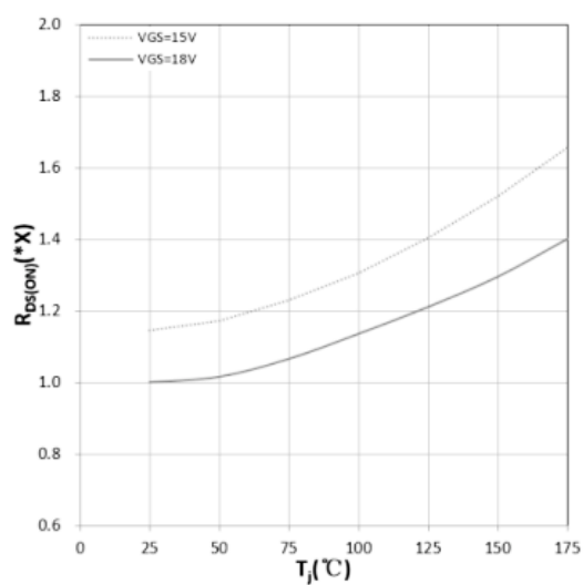
图 5 R_{DS(on)} 随 T_J 变化曲线
