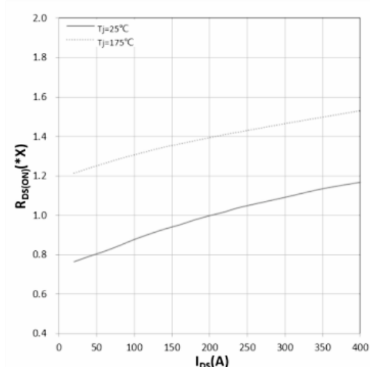
图 6 R_{DS(on)} 随 I_{DS} 的变化曲线
