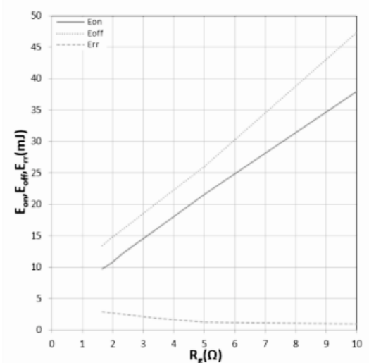
图 10 E_{on} , E_{off} , E_{rr} 随 R_g 的变化曲线
