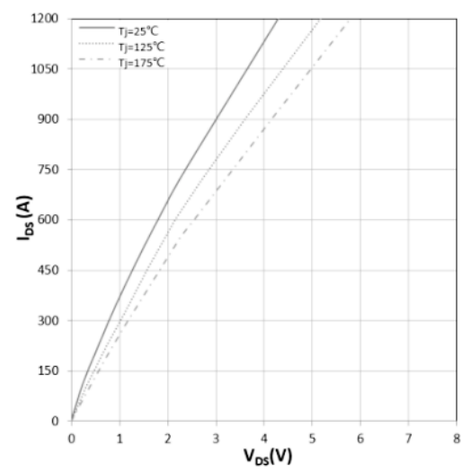
图 2 I_D 随 V_{DS} 的变化曲线
