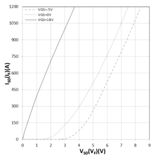
图 3 I_{SD} 随 V_{SD} 的变化曲线
