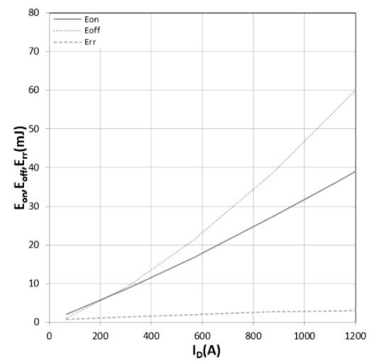
图 12 E_{on} , E_{off} , E_{rr} 随 I_{DS} 的变化曲线
