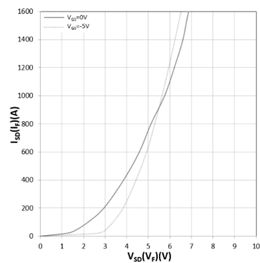
图 4 T_J=175^\circ\text{C} , 体二极管特性曲线
