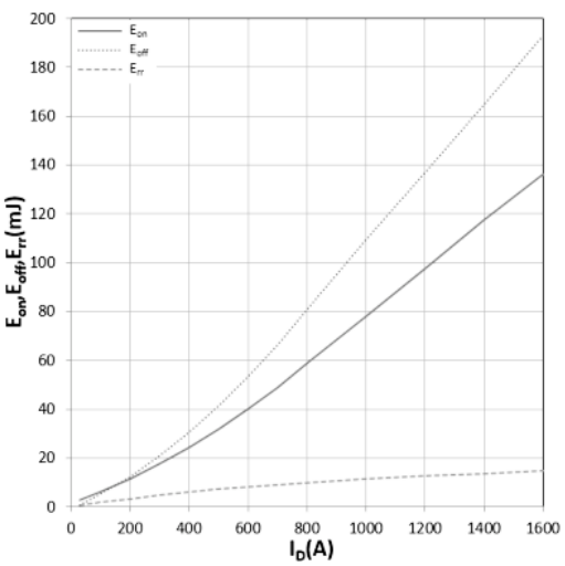
图 12 E_{on} , E_{off} , E_{rr} 随 I_{DS} 的变化曲线
