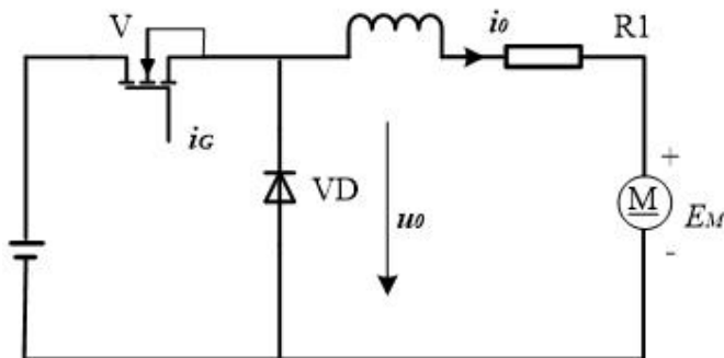
图 3 典型开关电路
