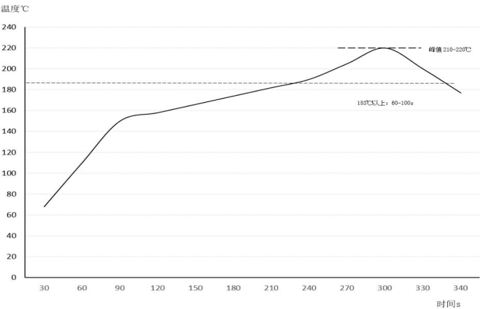
图 5 建议的回流焊曲线
