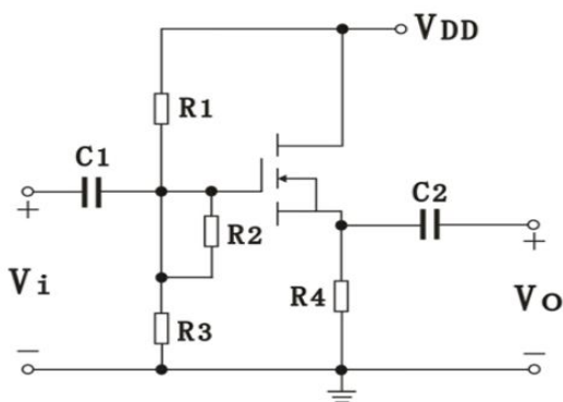
图 4 共漏极放大电路
