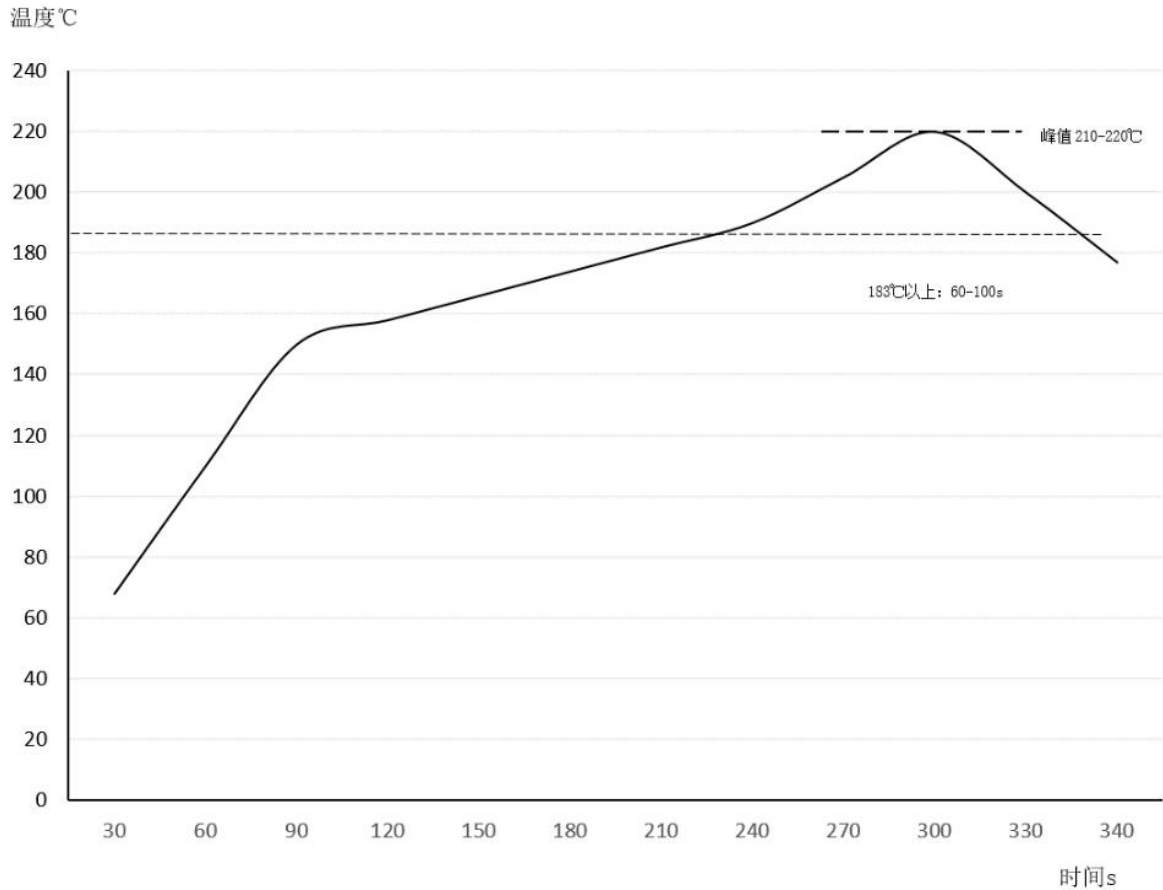
图 11 建议的回流焊曲线
