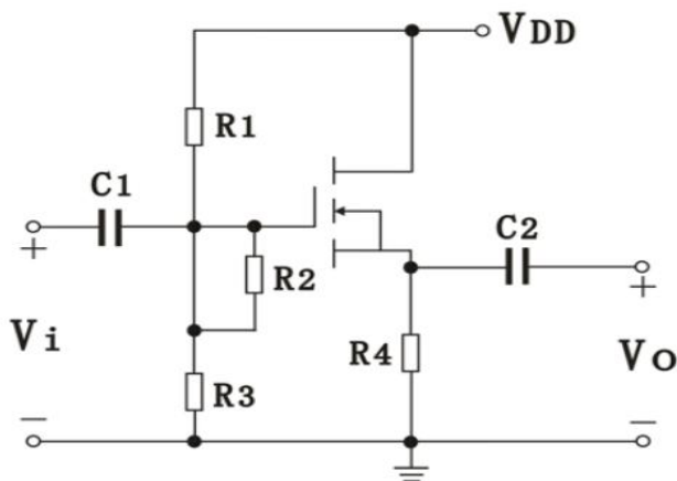
图 10 共漏极放大电路
