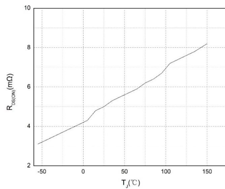
图 2 R_{DS(on)} - T_J 特性曲线
