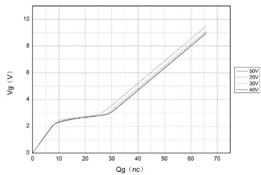
图 4 V_{GS} - Q_g 特性曲线
