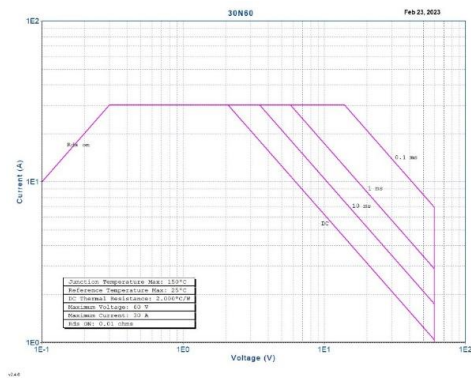
图 5 安全工作区曲线
