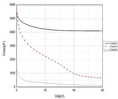
图 3 电容曲线
