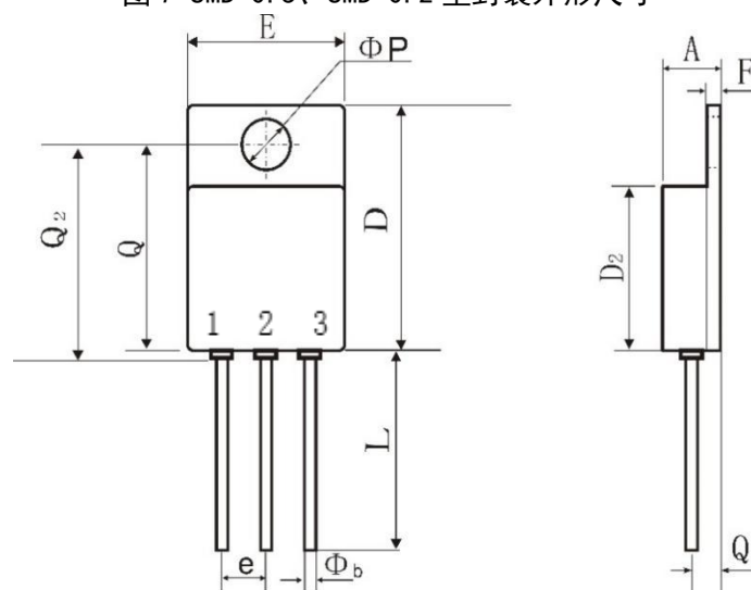
图 7 SMD-0.5、SMD-0.2 型封装外形尺寸
