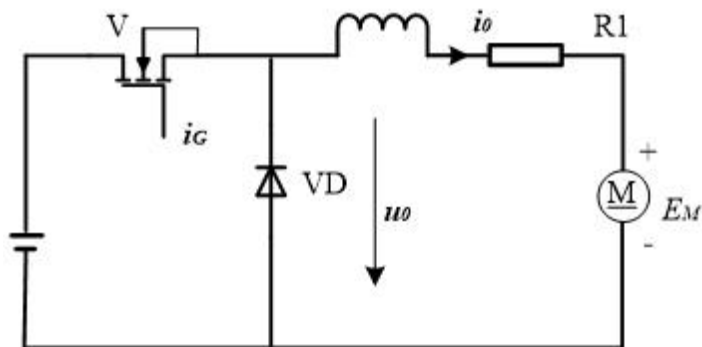
图 9 典型开关电路
