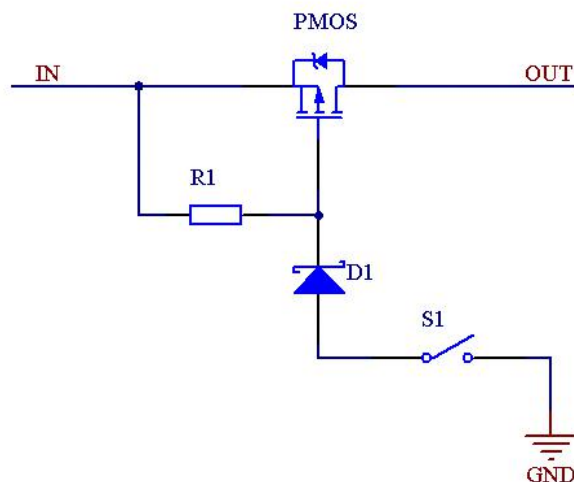
图 3 典型开关电路
