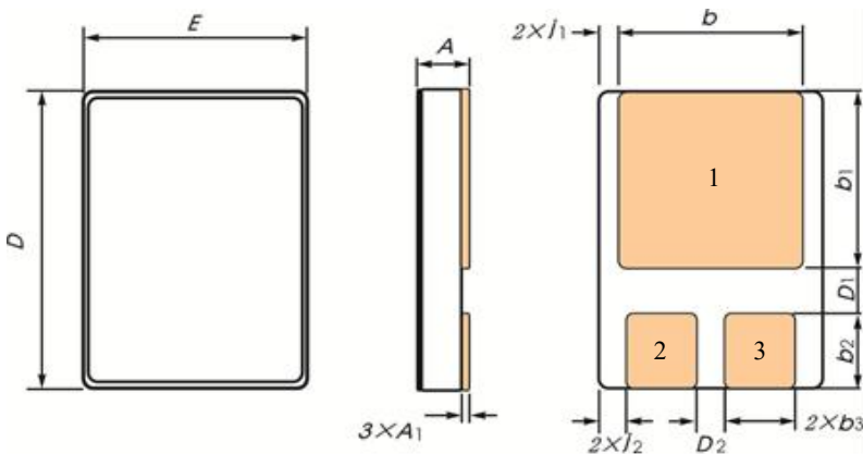
图 1 T0-257 外形尺寸
