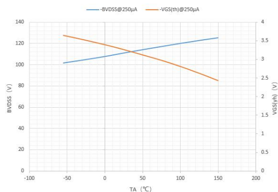
图 2 漏源击穿电压、阈值电压特性曲线
