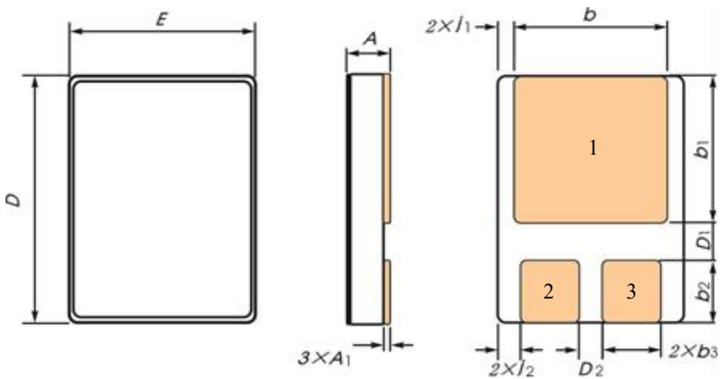
图5 T0-257 外形尺寸
