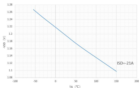
图 3 体二极管正向压降特性曲线
