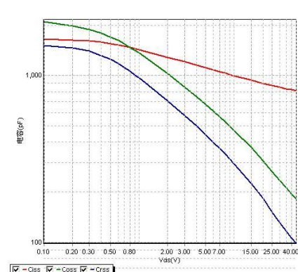
图 4 电容特性曲线
