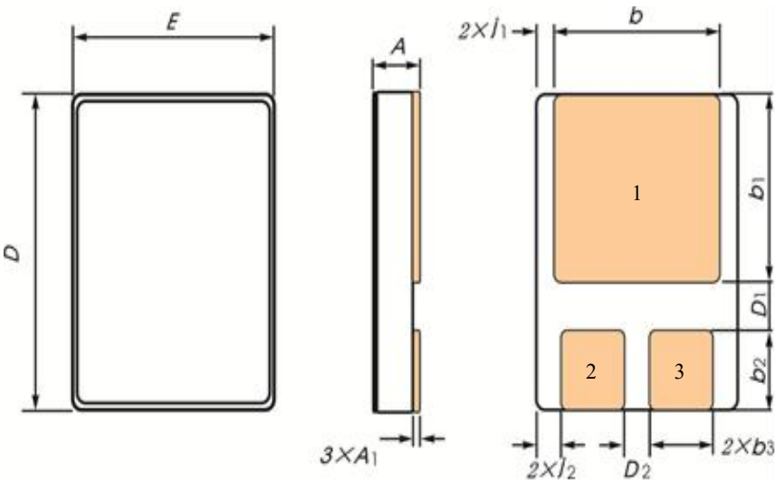
图 1 T0-254 外形尺寸
