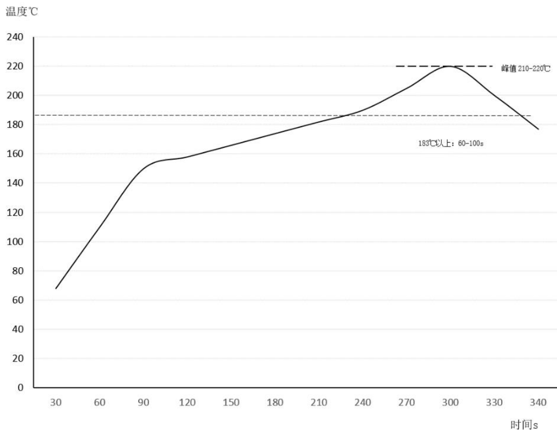
图 7 建议的回流焊曲线
