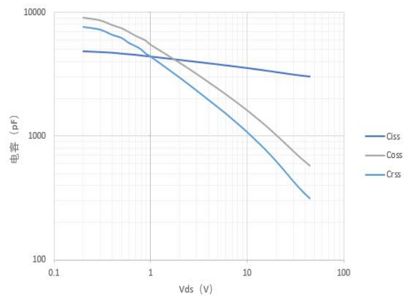
图4 电容特性曲线
