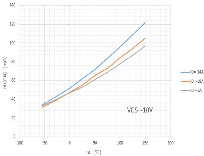
图 1 导通电阻特性曲线
