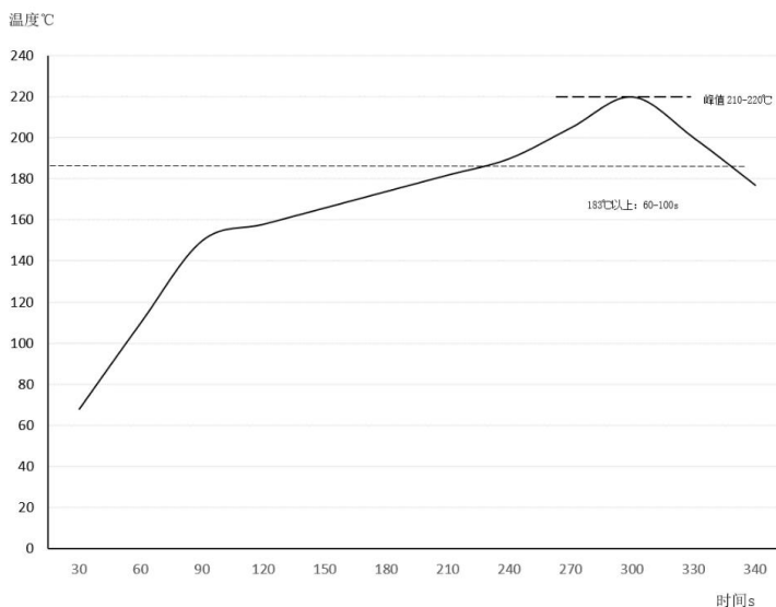
图 8 建议的回流焊曲线
