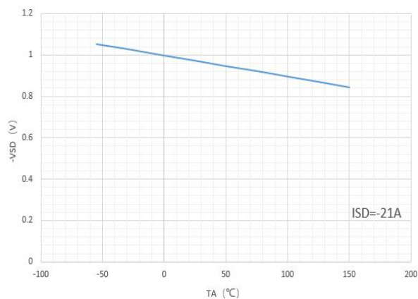
图3 体二极管正向压降特性曲线
