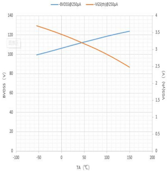
图 2 漏源击穿电压、阈值电压特性曲线
