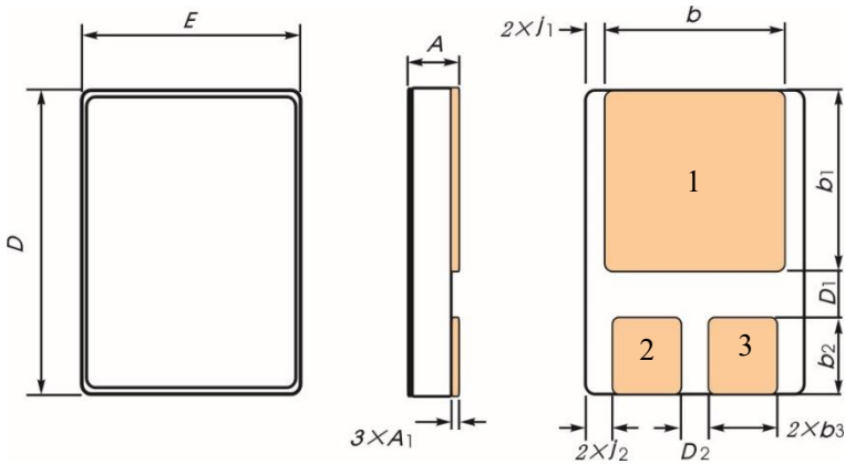
图 7 SMD-2 外形尺寸
