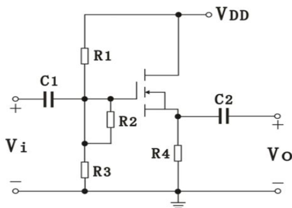
图 10 共漏极放大电路
