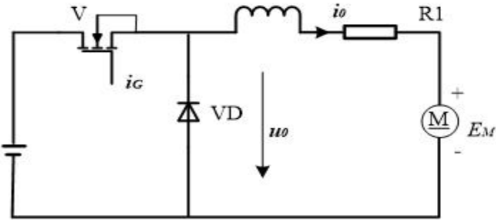
图 9 典型开关电路
