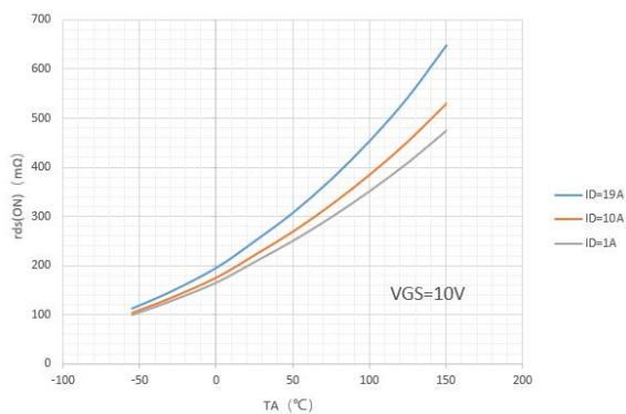
图 1 导通电阻特性曲线
