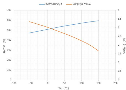
图 2 漏源击穿电压、阈值电压特性曲线
