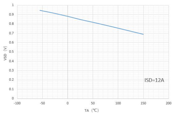
图 3 体二极管正向压降特性曲线
