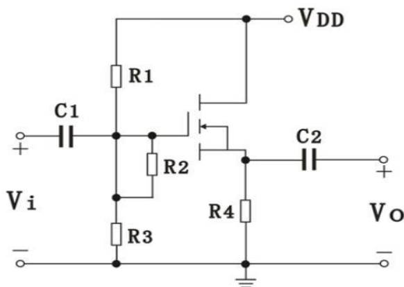
图 3 共漏极放大电路
