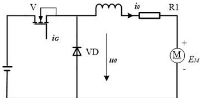
图 2 典型开关电路
