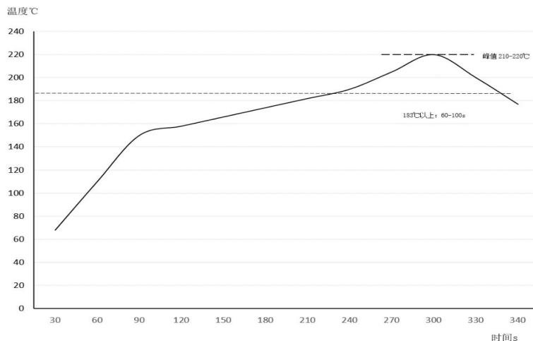
图 4 建议的回流焊曲线
