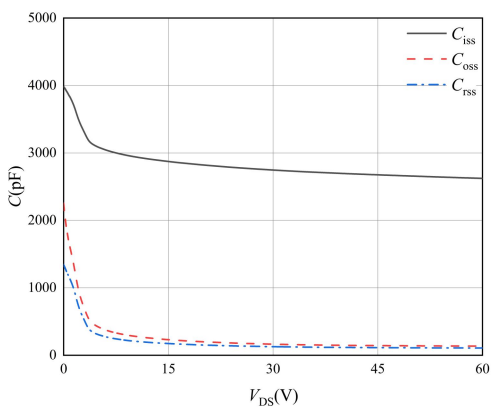
图 5 C-V_{DS} 特性曲线
