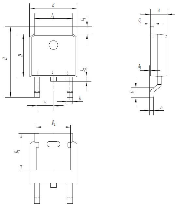
引出端：1-栅极 G，2-漏极 D，3-源极 S
