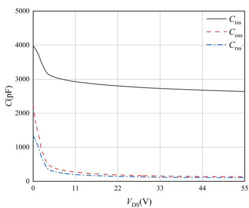
图 5 C-V_{DS} 特性曲线
