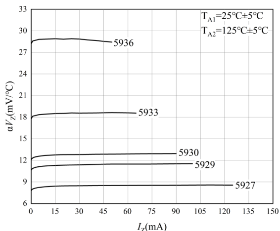
图 3 温度漂移特性曲线
