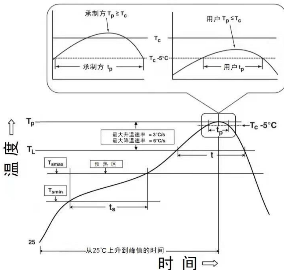
图 15 回流温度-时间分布图
