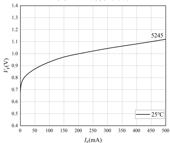
图 3 正向特性曲线-3
