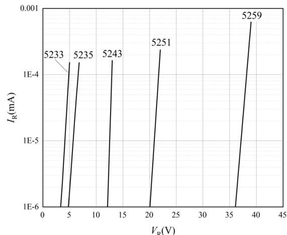
图 6 反向特性曲线-2
