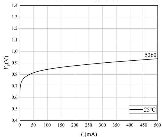
图 4 正向特性曲线-4
