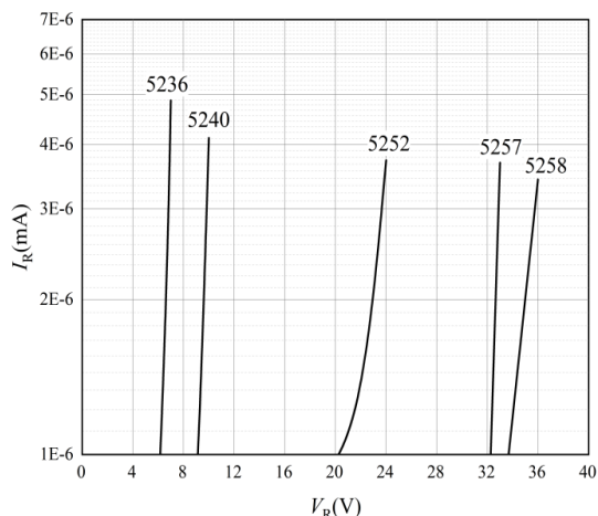
图 7 反向特性曲线-3
