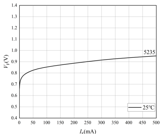
图 2 正向特性曲线-2
