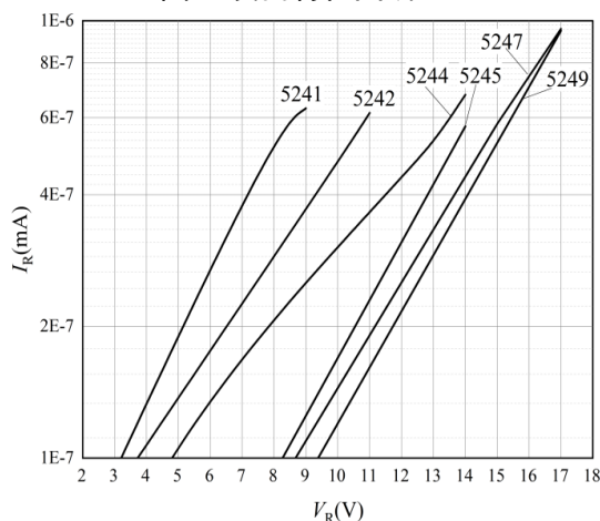
图 9 反向特性曲线-5
