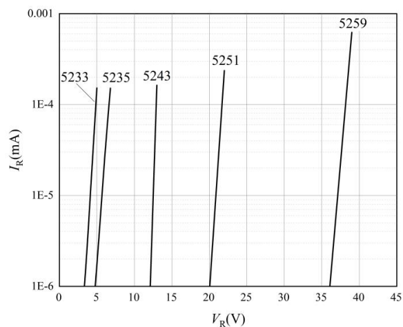
图 6 反向特性曲线-2
