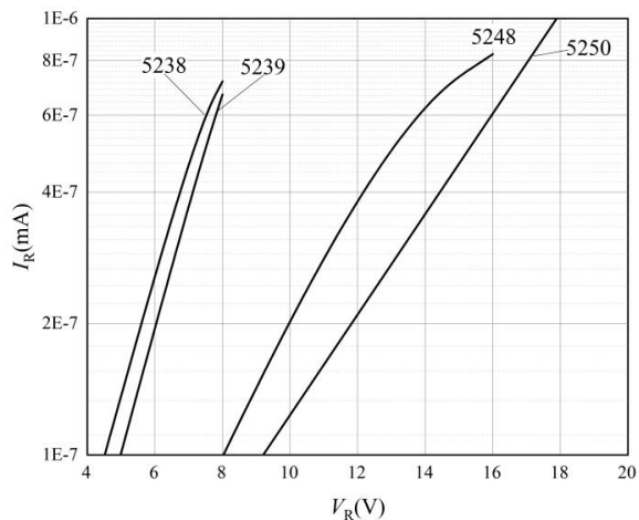
图 8 反向特性曲线-4
