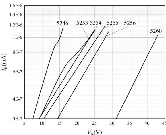
图 10 反向特性曲线-6
