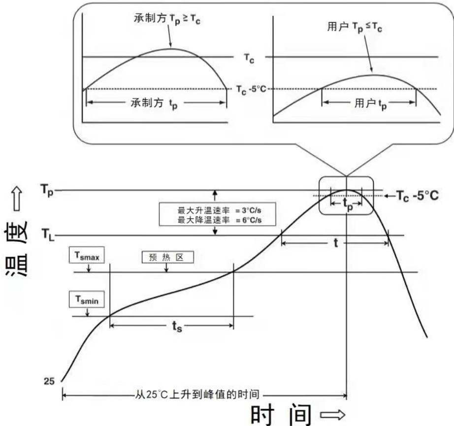
图 15 回流温度-时间分布图
