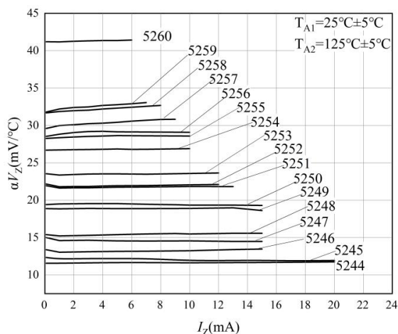
图 12 温度漂移特性曲线-2
