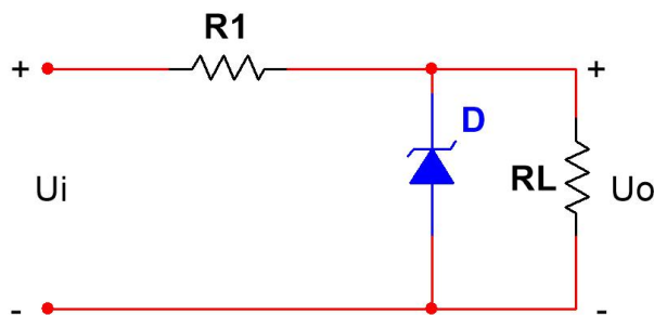
图 14 典型的应用连接图
