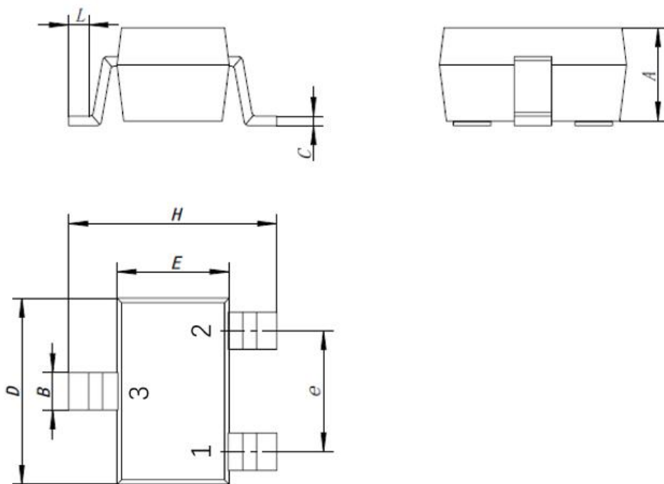
引出端：1-栅极 G，2-源极 S，3-漏极 D
