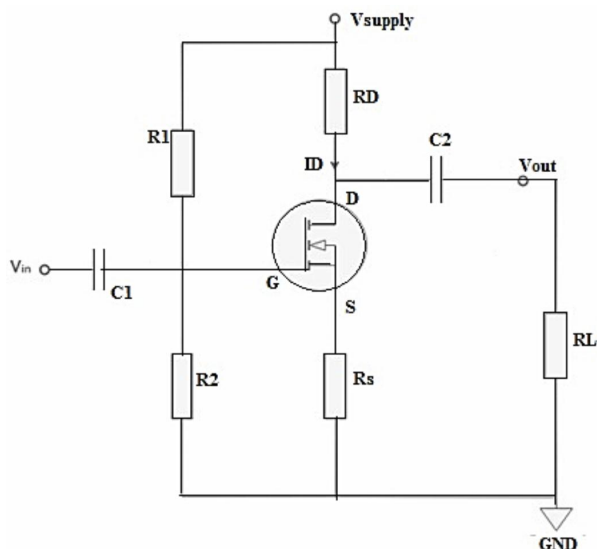
图 3 典型放大电路
