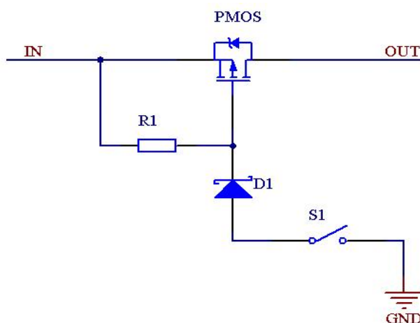
图 2 典型开关电路
