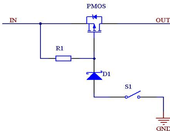
图 2 典型开关电路
