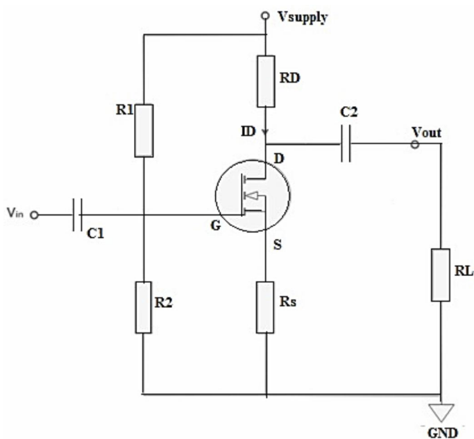
图 3 典型放大电路
