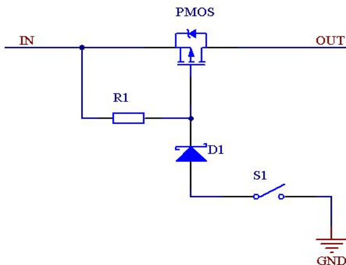
图 2 典型开关电路
