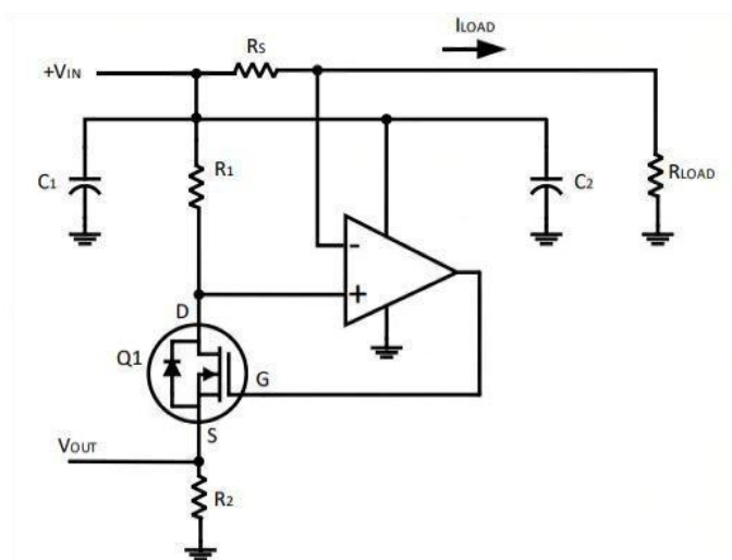
图 2 耗尽型场效应管开关电路
