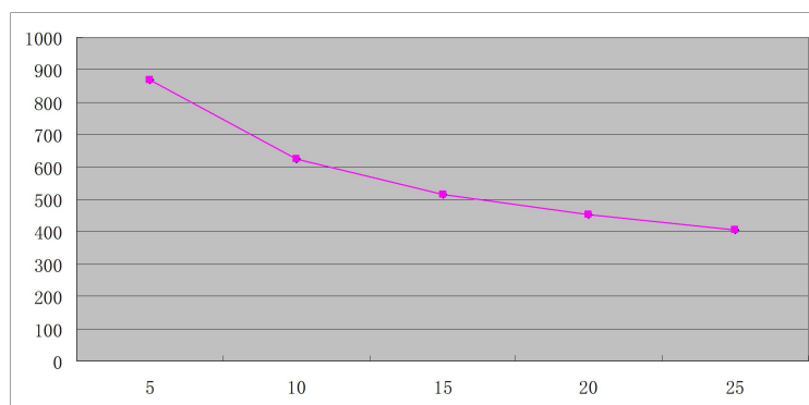
图 3 C_{tot} — V_R 特性曲线
