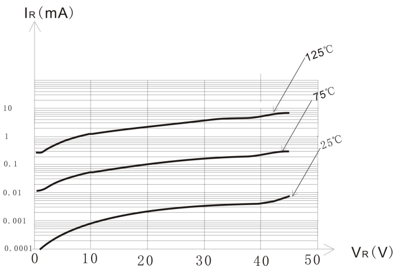
图 1 I_R — V_R 特性曲线
