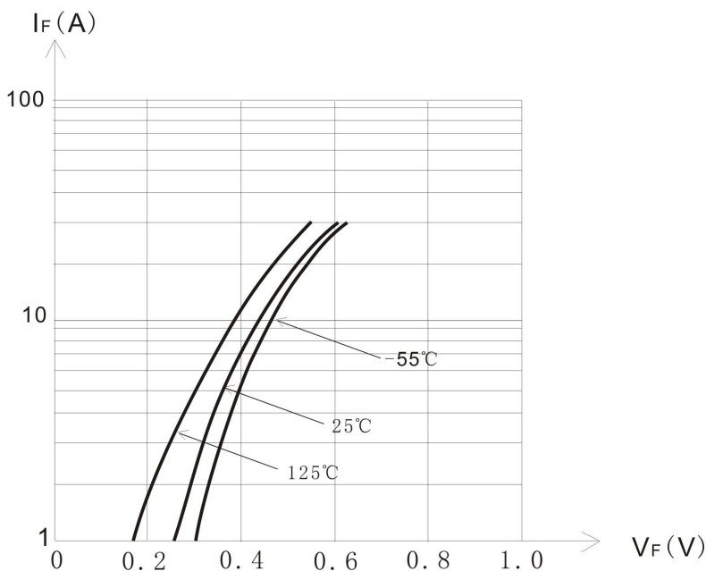
图 2 V_F — I_F 特性曲线
