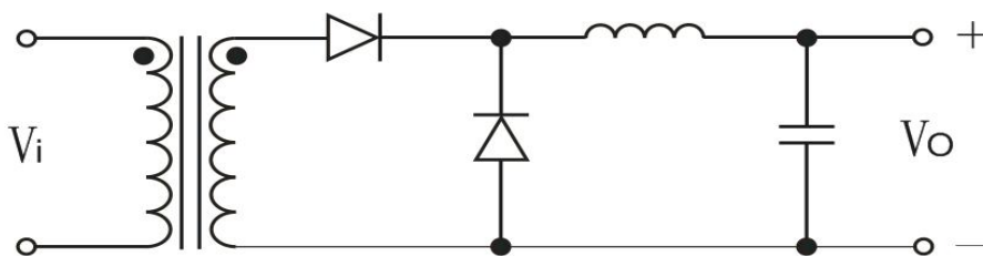
图 7 整流加续流电路
