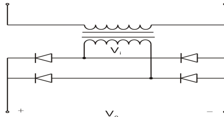
图 6 单相全波整流电路
