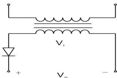
图 5 单相半波整流电路
