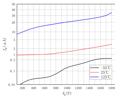
图 2 反向特性曲线
