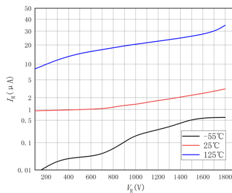
图 2 反向特性曲线
