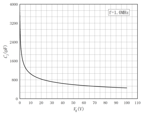
图 3 结电容特性曲线
