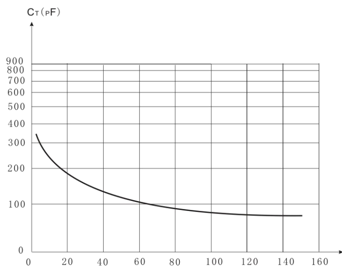
图 3 C_T - V_R 特性曲线
