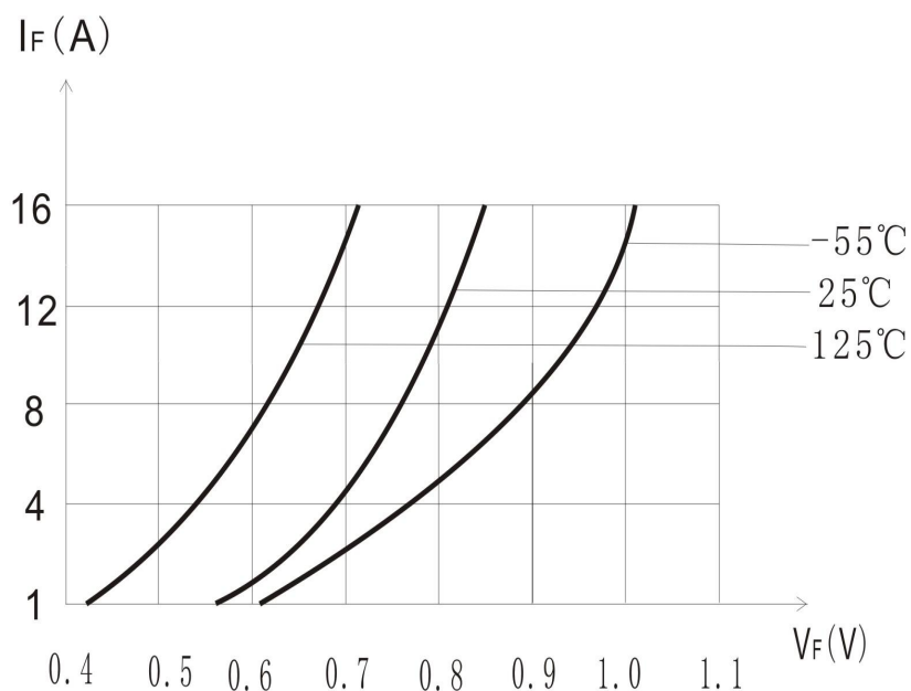
图2 V_F - I_F 特性曲线
