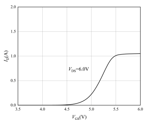
图 2 转移特性曲线
