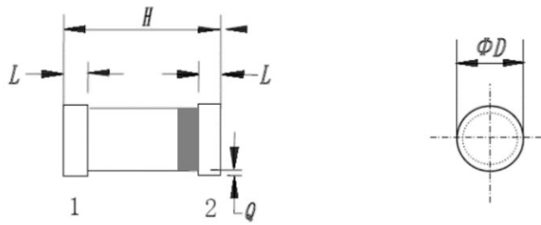
器件 1 端为正极，2 端（带色环）为负极
