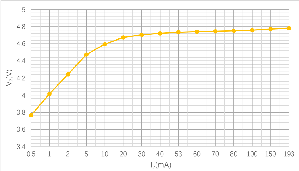
图 1 V_Z — I_Z 特性曲线
