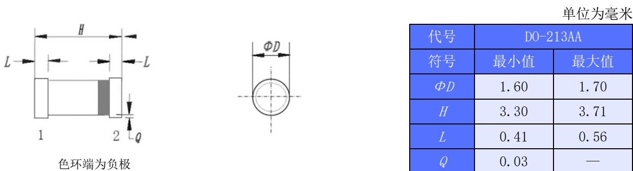
图 2 DO-213AA 外形尺寸
